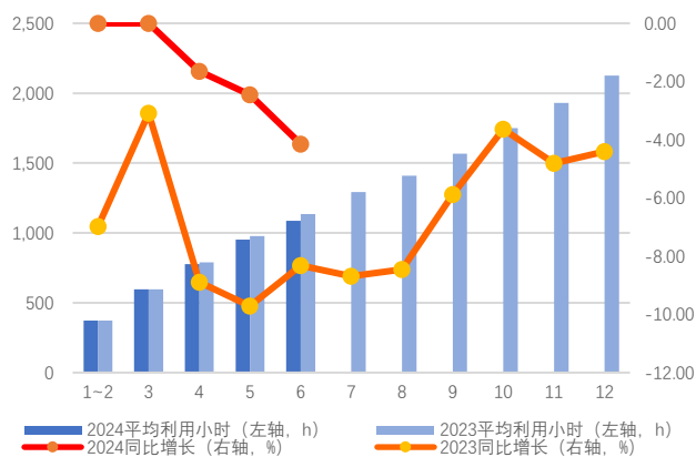
图 50: 风电发电设备平均利用小时数
