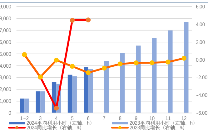
图 49: 核电发电设备平均利用小时数
