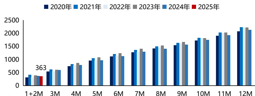
图13：风电累计利用小时数月度变化情况（小时）
