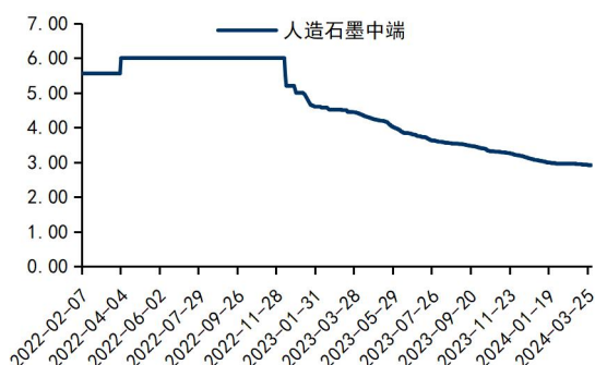
图17: 人造石墨负极价格走势（万元/吨）
