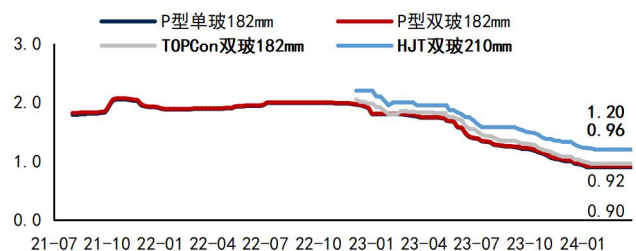
图24: 组件价格 (元/W)
