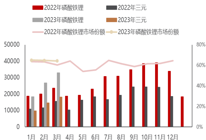
图18：22-23 年 3 月磷酸铁锂和三元电池产量(MWh)
