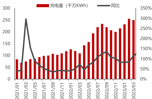
图26：21-23 年 3 月公共类充电设施充电电量情况 (KWh)
