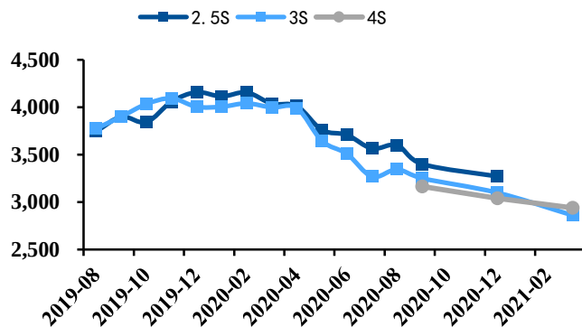
图4: 风机投标价格持续下降 (单位: 元/kW)
